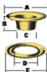
Grommets&Washers
